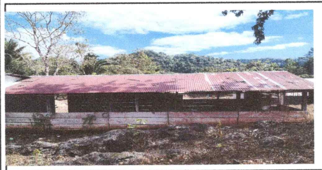
Foto 5: se observa el deterioro del techo del modulo 3
